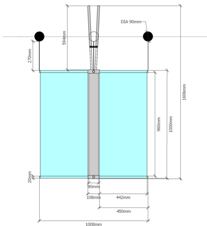
Figura 1: Rappresentazione schematica di un drifter CODE con le misure in mm.
