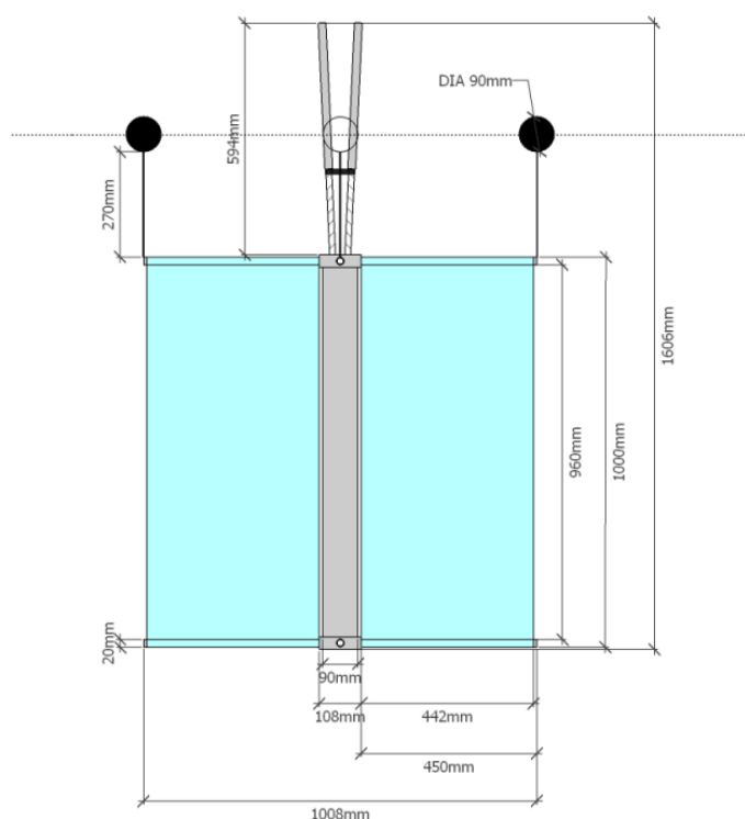
Figura 1 - Rappresentazione schematica di un drifter CODE
